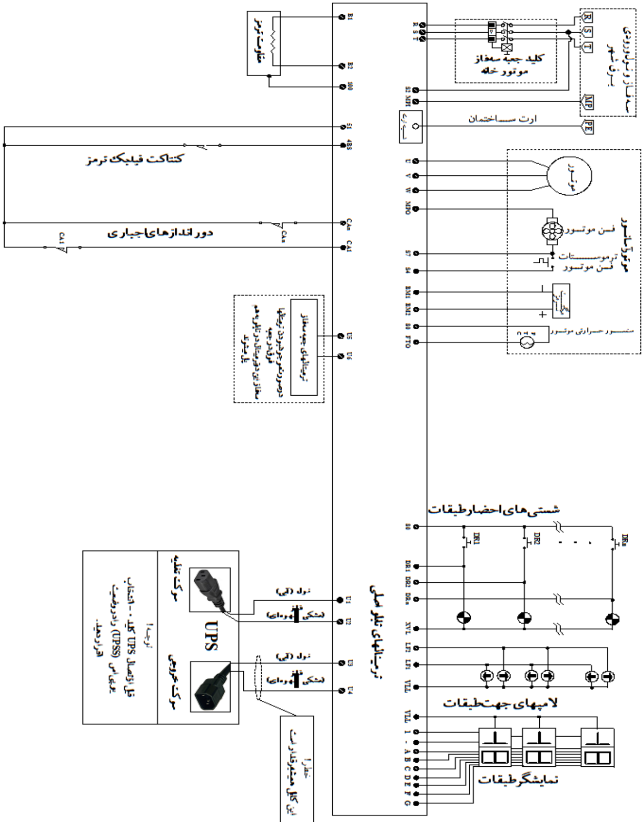
ضمیمه E: نقشه سیم کشی تابلو فرمان:
