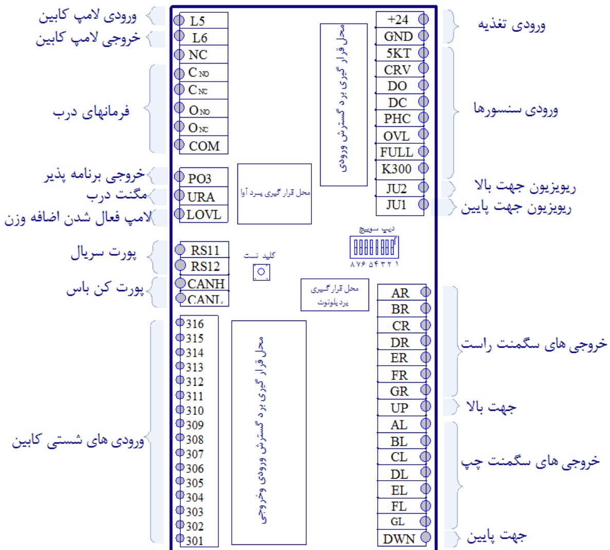
شمای برد کارکدک
