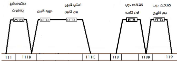
ترمینال‌های برد Carcodec S05-05
