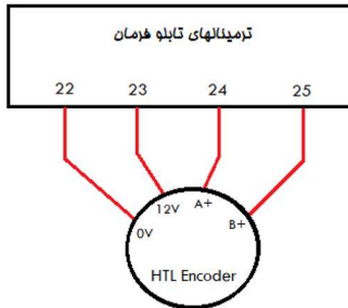
۵ . ۳ . ۲ . ۳ . ۱ . ۳ . ۵ . انکودر SINCOS موتور گیرلس ( مانند ERN1387 و ERN487 )
